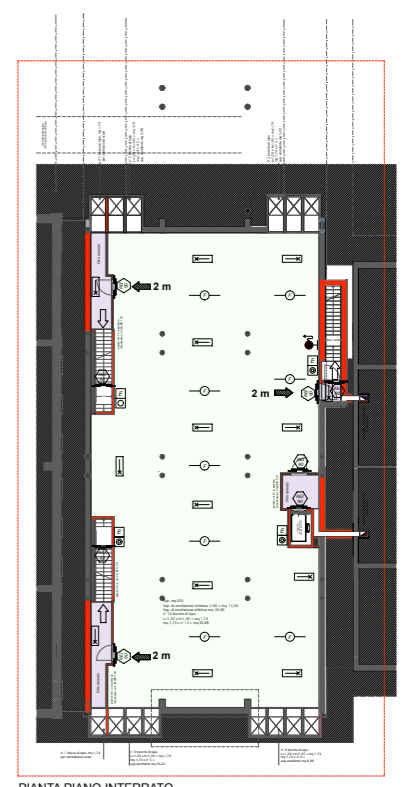
PIANTA PIANO INTERRATO
